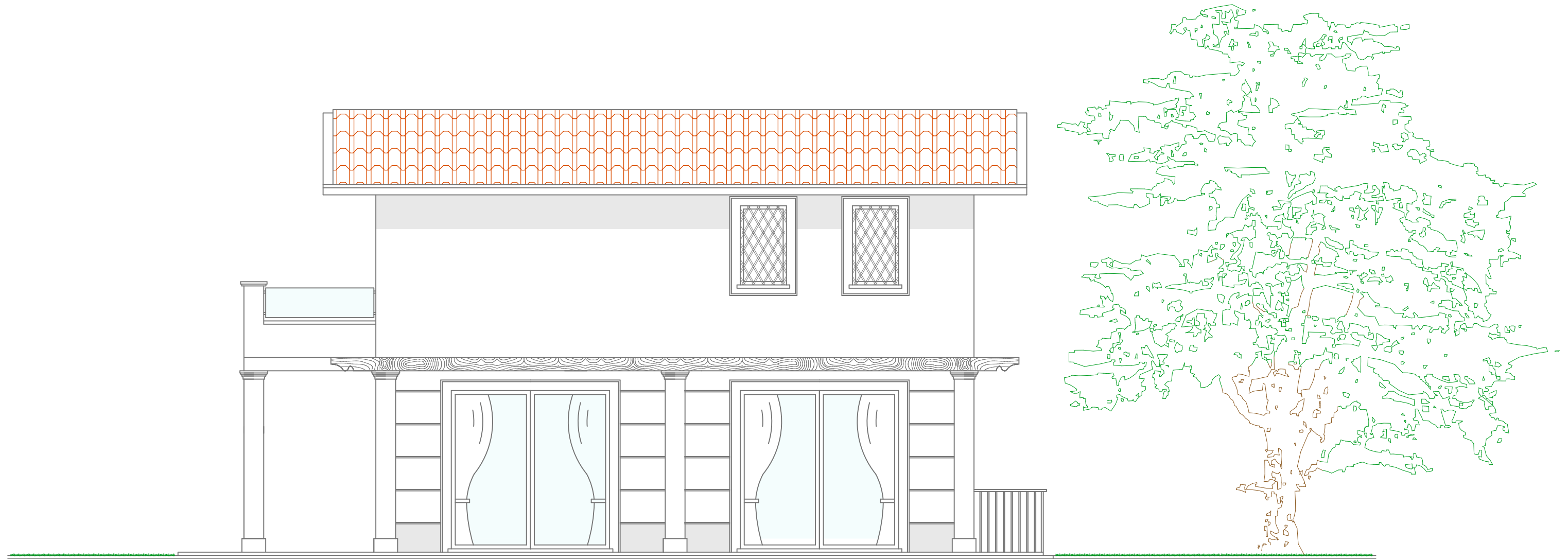
Prospetto Lato Mare
